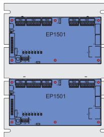
(2) EP1501 PCB
